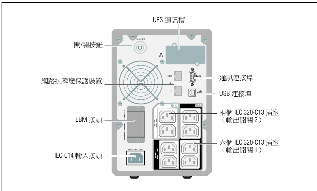
圖 6. 1000W，230V 後面板
