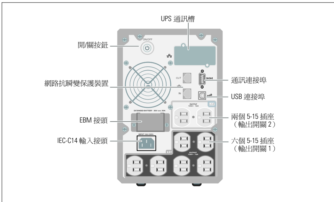
圖 5. 1000W，120V 後面板
