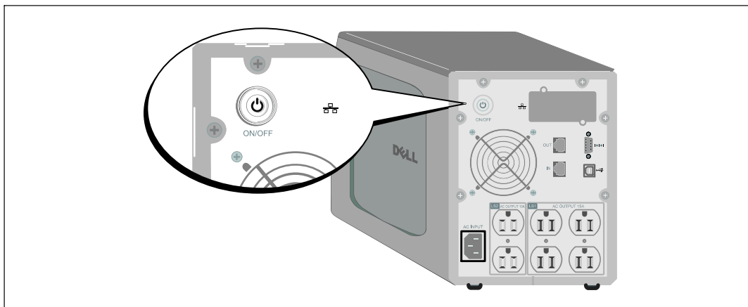
圖 18. 啟動 UPS
